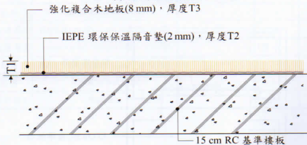
(b)A-A'剖面示意圖
